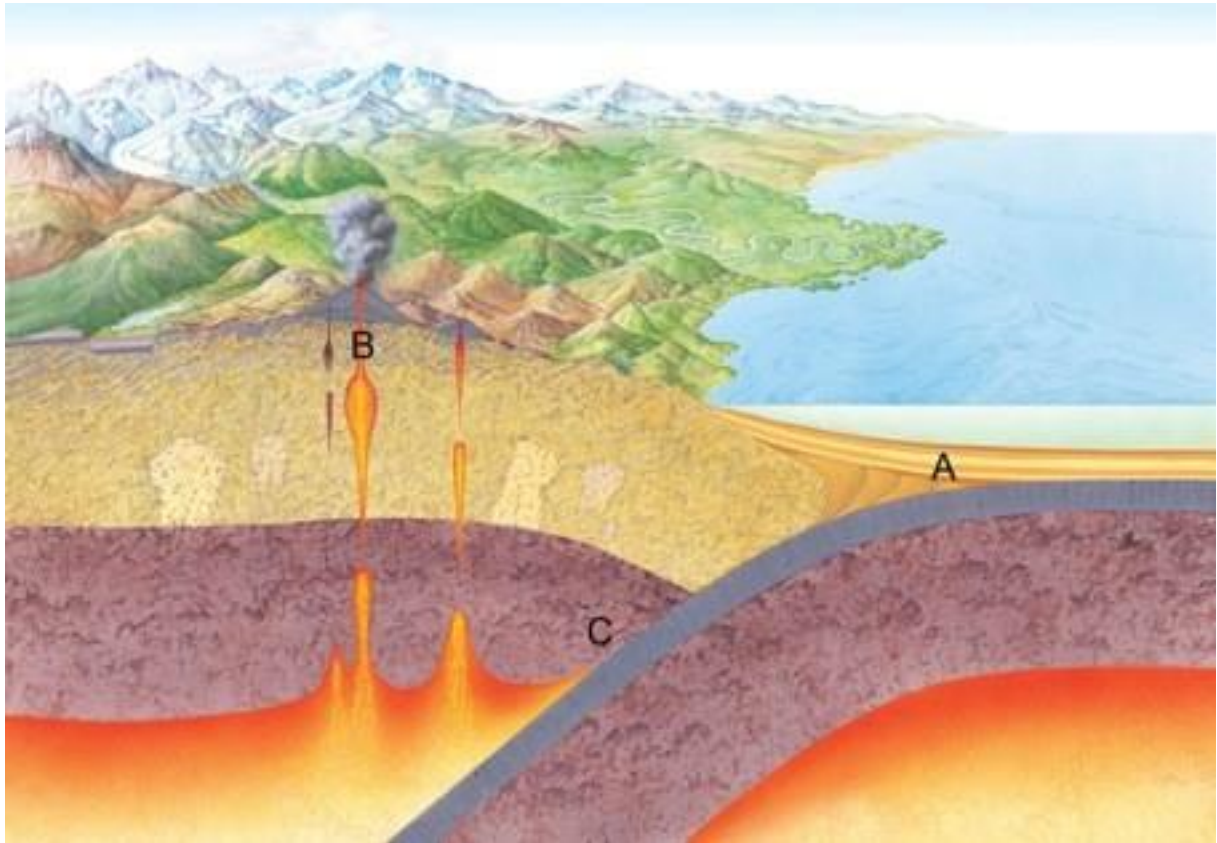
Նկ A 1: Լեռնակազմություն /ապարների ձևավորումը/
